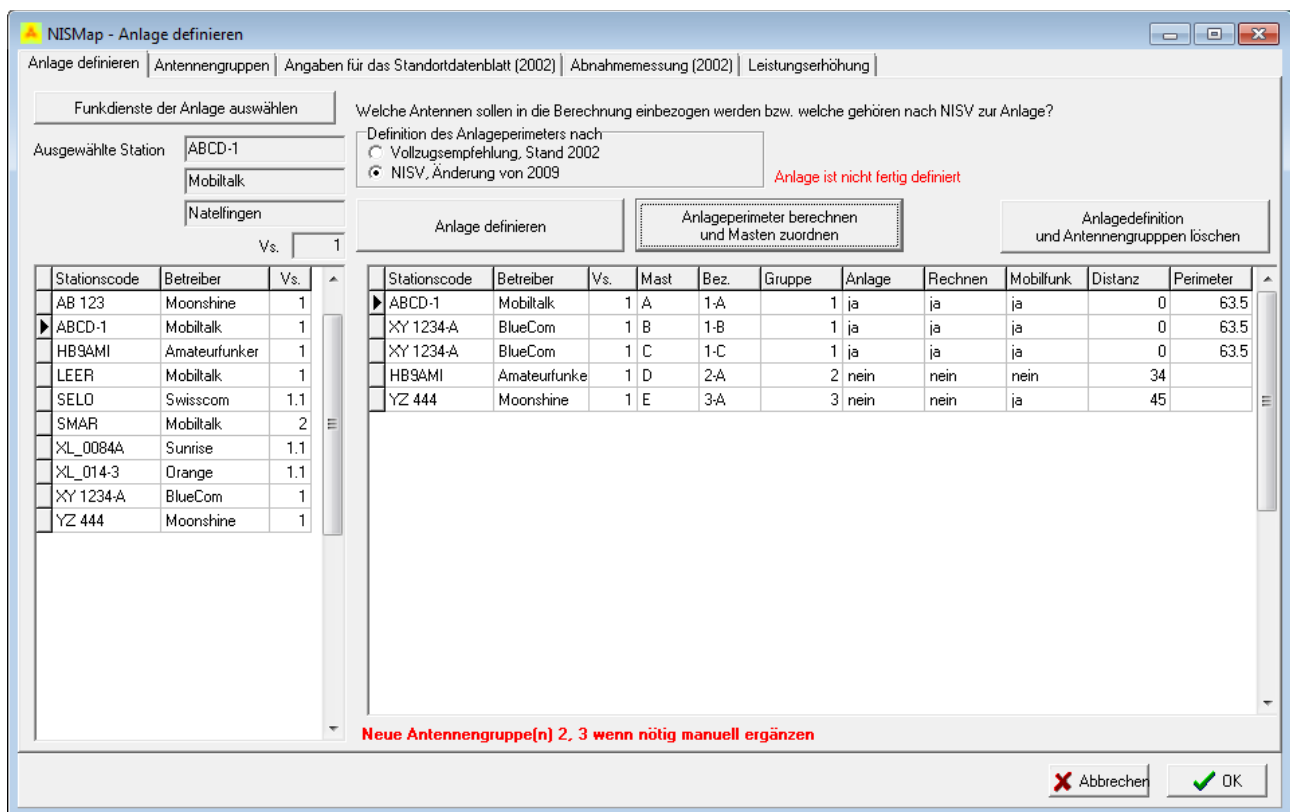
Abbildung 13: Anlagedefinition mit Antennengruppen (NISV, Änderung 2009).
