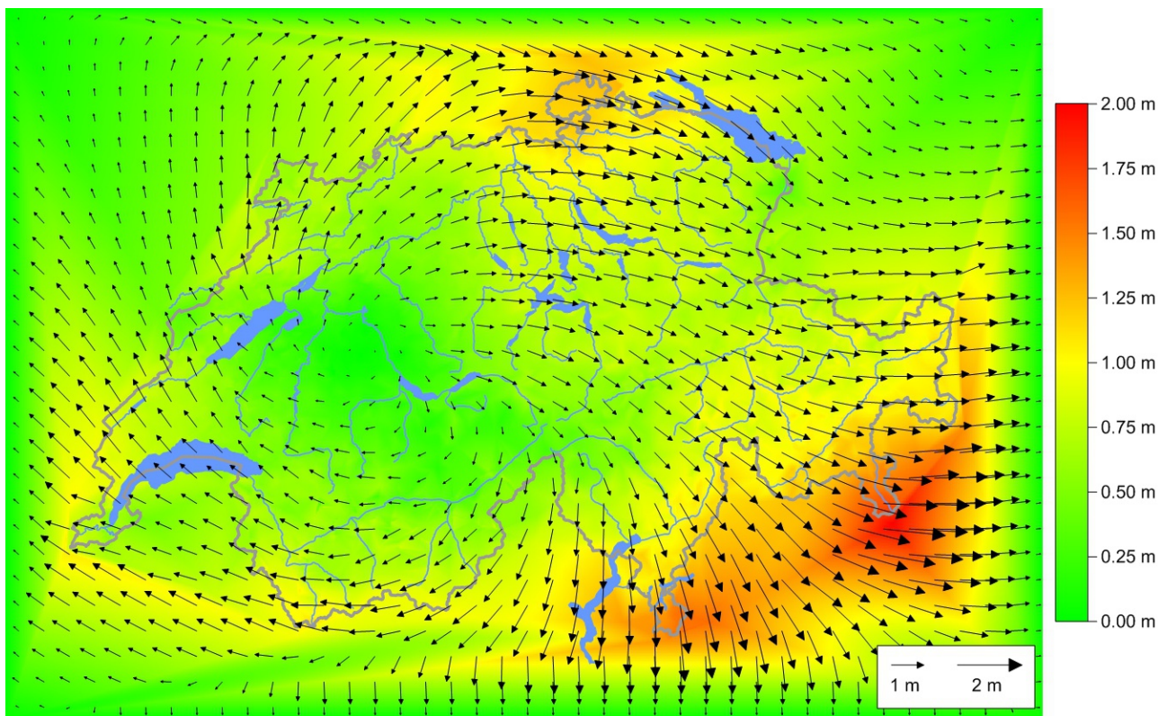
Abbildung 52: Verzerrung zwischen LV03 und LV95 (abgesehen von der Verschiebung des Ursprungs). Der Betrag der Verzerrung ist durch die Farbe angezeigt, die Pfeile zeigen zusätzlich zum Betrag auch die Richtung der Verschiebung.
